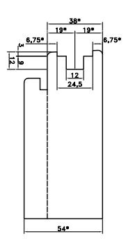
VOORBEELD DETAIL 1: deurdikte 38 / 54 mm T-groef
