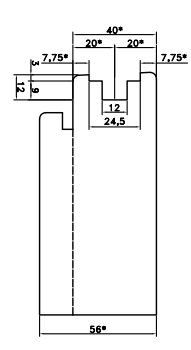
VOORBEELD DETAIL 2: deurdikte 40 / 56 mm T-groef
